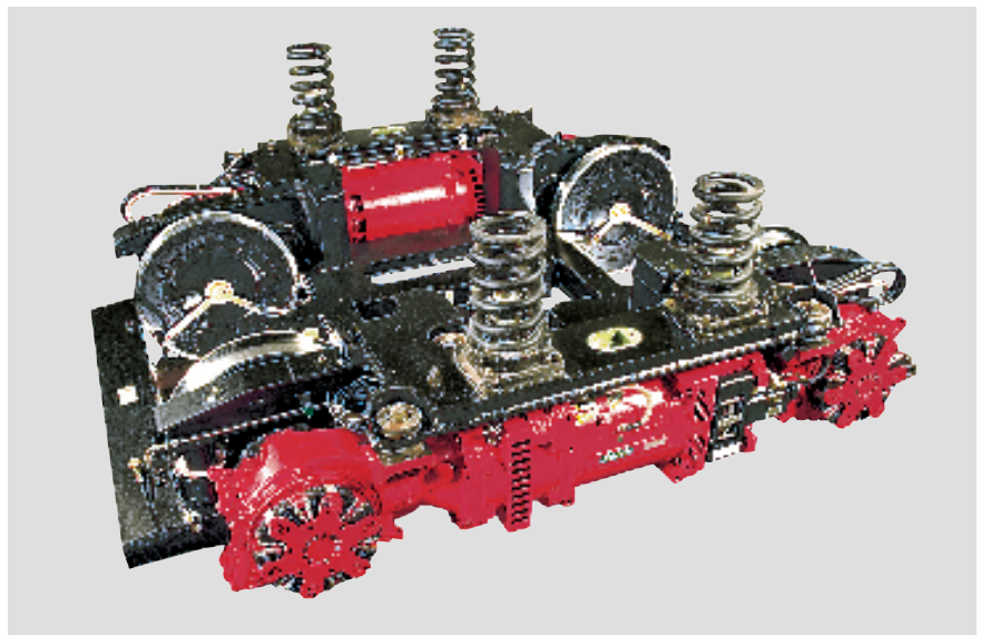
COMBINO-Triebfahrwerk
