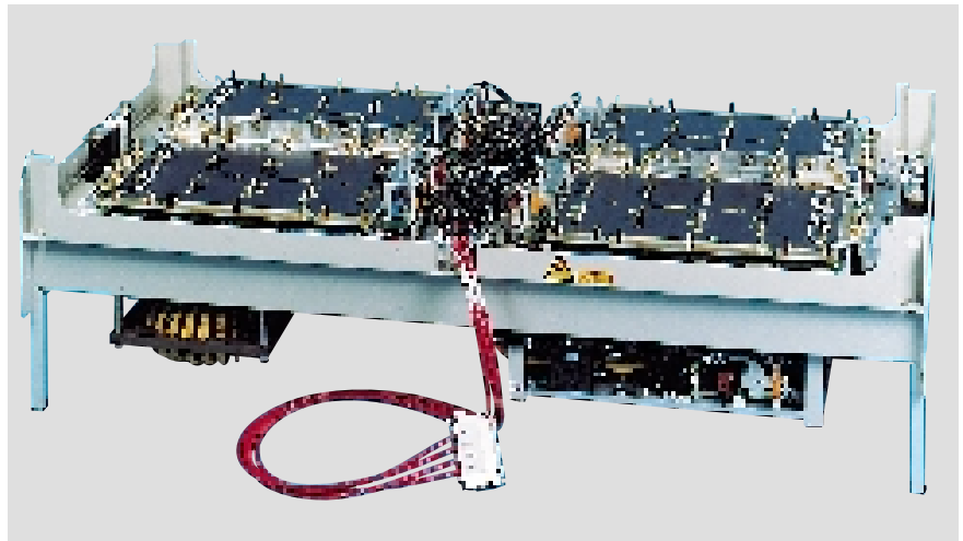
COMBINO-Traktionsstromrichter
