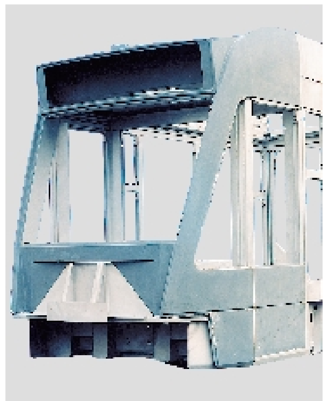
Rohbau des Triebmoduls mit GfK-Fahrzeugkopf
