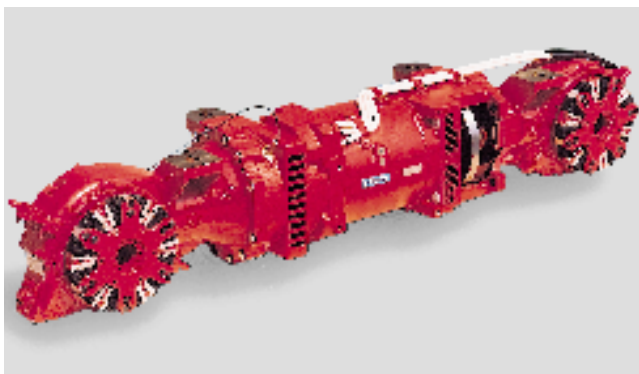
COMBINO-Antriebsaggregat
